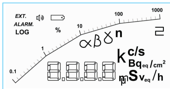
Radiagem 2000 Display.
